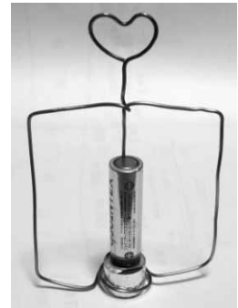
Fig. 2 Faraday’s Motor.
